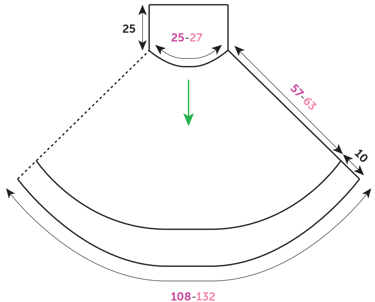
Tekening, maten in cm
